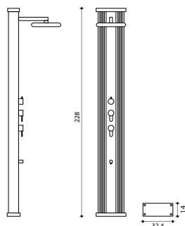
Rociador de ducha anti-cal integrado
